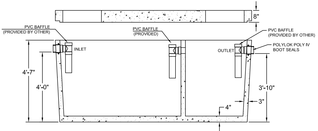
SECTION A-A
