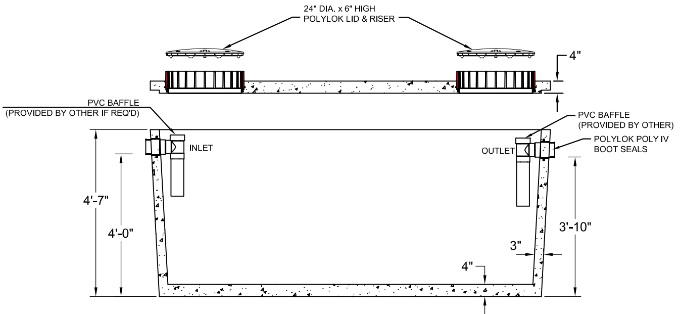
SECTION A-A
